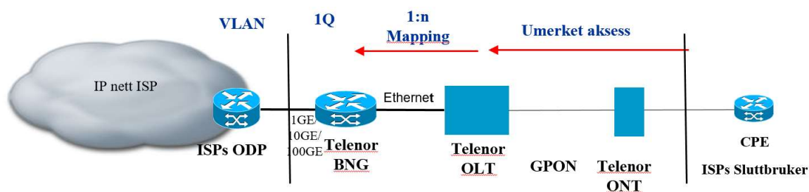
Figur 1 - Referansefigur VULA på Shared VLAN
