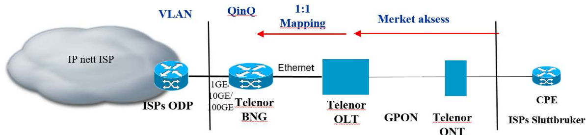
Figur 2 - Referansefigur VULA på Dedicated tagged VLAN
